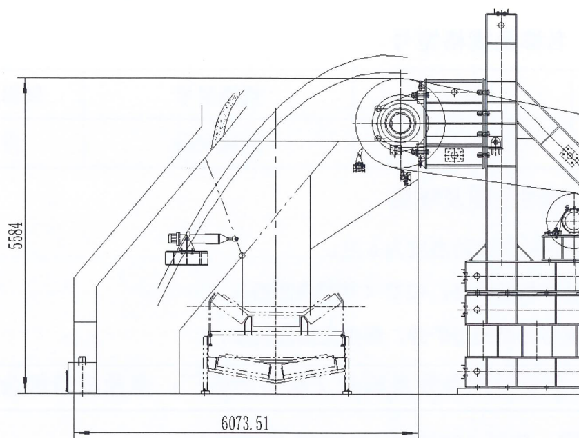
图 1 订货示意图，宽度 2500mm
