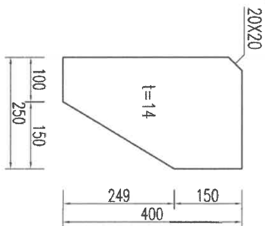
详图 5 (桩顶肋板)
