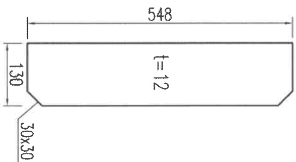
详图 12
