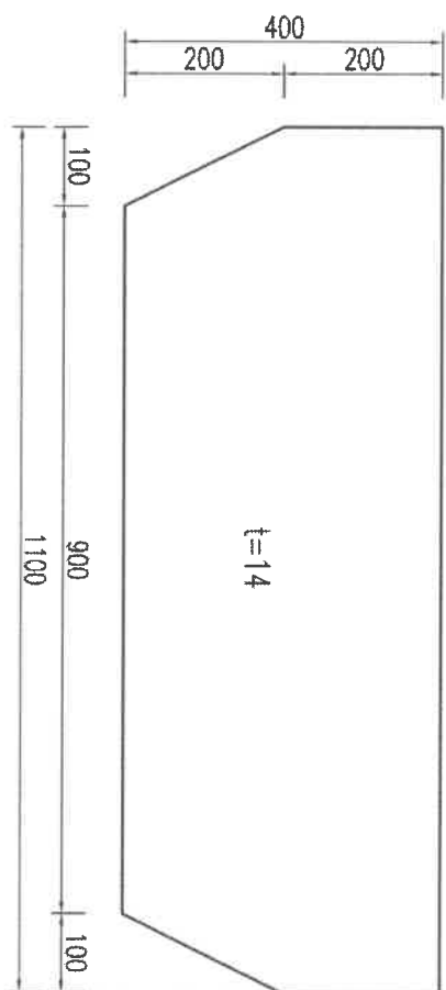
详图 2 (件 2)
