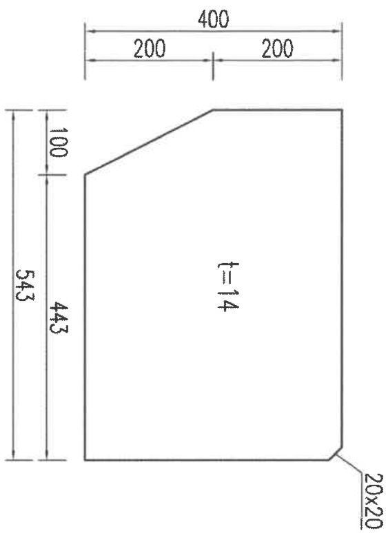
详图 3 (件 3)
