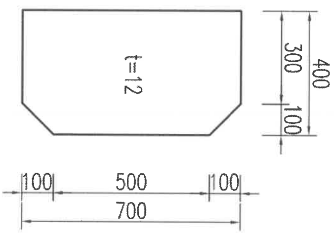
详图 16 (节点板)
