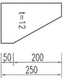
详图 11
