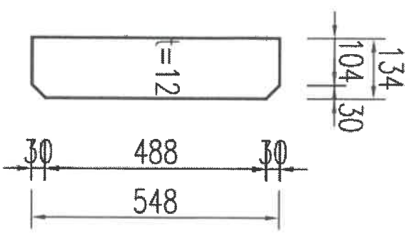
详图 14 (主横梁加劲板 1) 详图 15 (主横梁加劲板 2)
