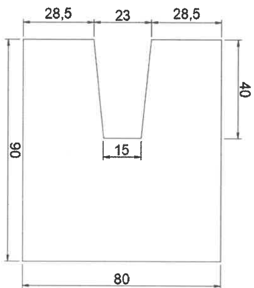
详图 1 (贝雷上卡扣)
