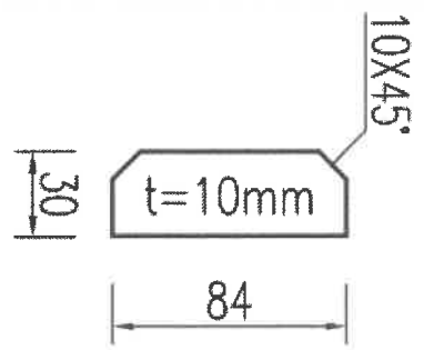
详图 18 (劲板)
