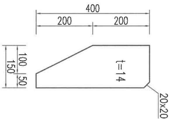
详图 4 (件 4)
