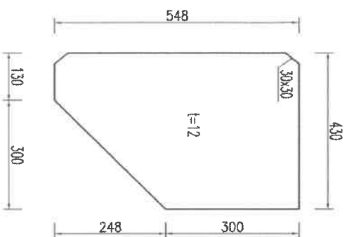
详图 9 (主横梁肋板 2)
