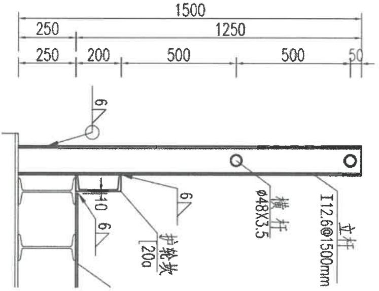
详图 7 (栏杆立杆需要开孔)
