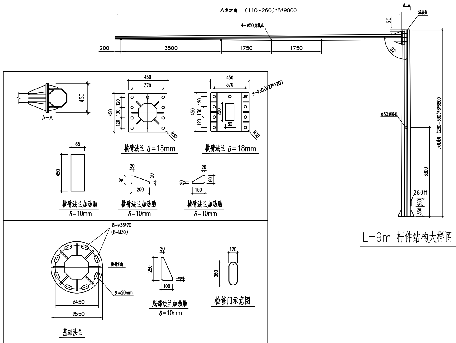
H6.8L9米八角电警杆
