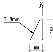
底部法兰加劲肋
