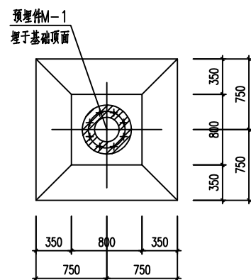
基础平面图
