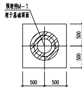
基础平面图
