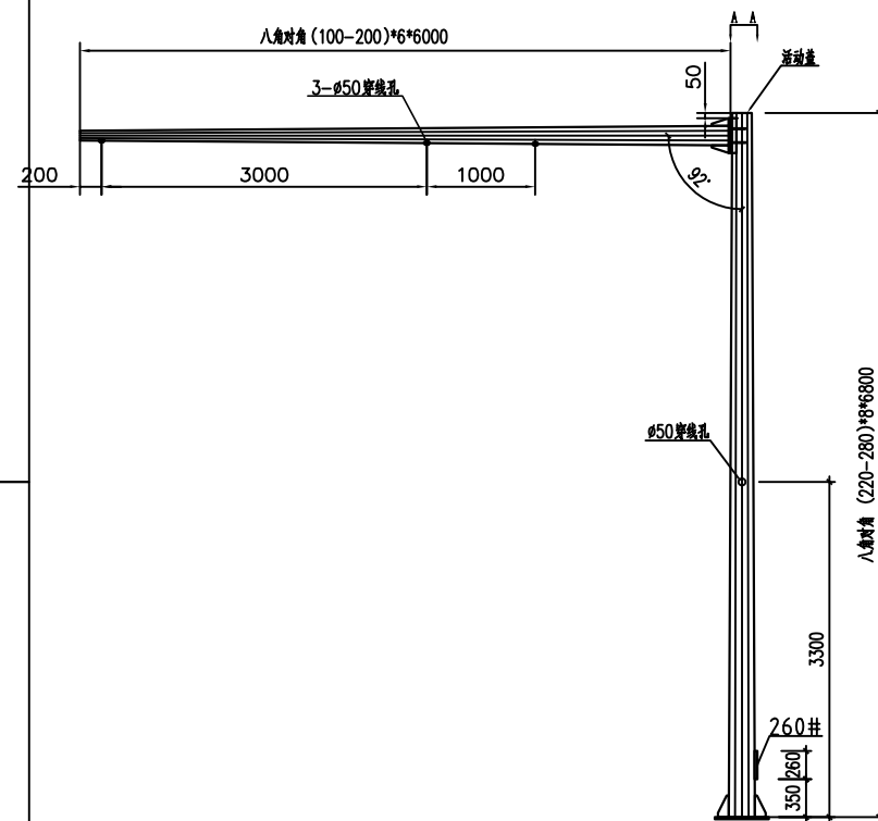
L=6m 杆件结构大样图
