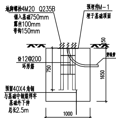
基础立面图
