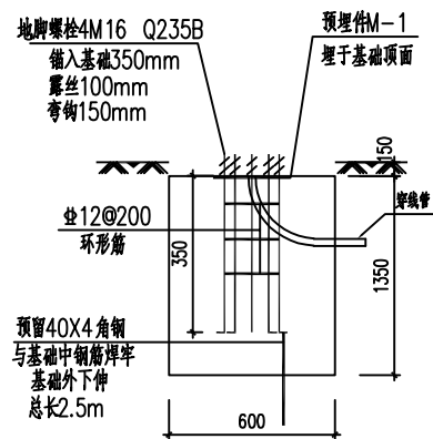
基础立面图
