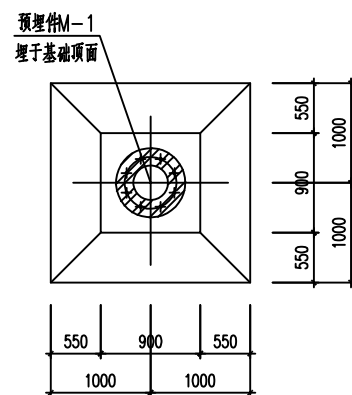
基础平面图
