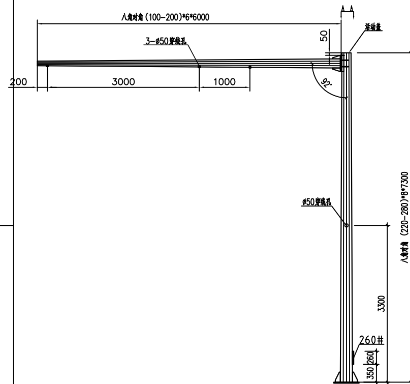
L=6\text{m} 杆件结构大样图
