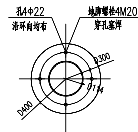
M-1 1:25 预埋钢板厚度为16mm
