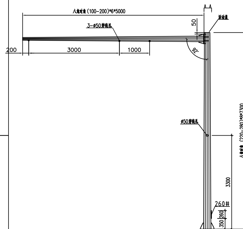
L=5m 杆件结构大样图
