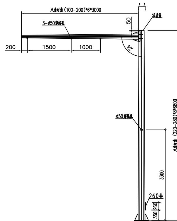
L=3m 杆件结构大样图
