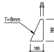
底部法兰加劲肋
