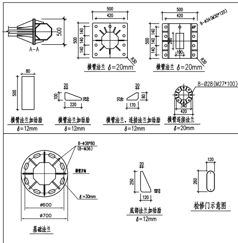
H6. 8L14米八角电警杆
