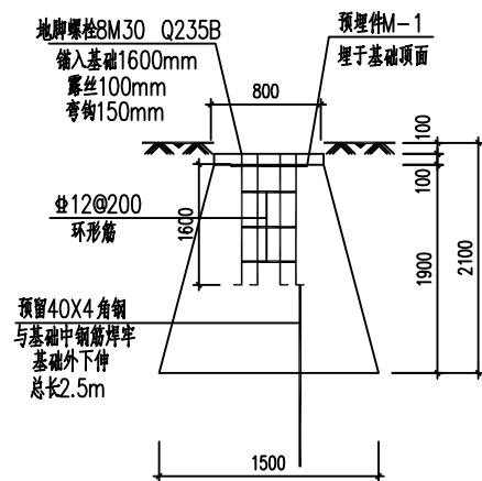
基础立面图
