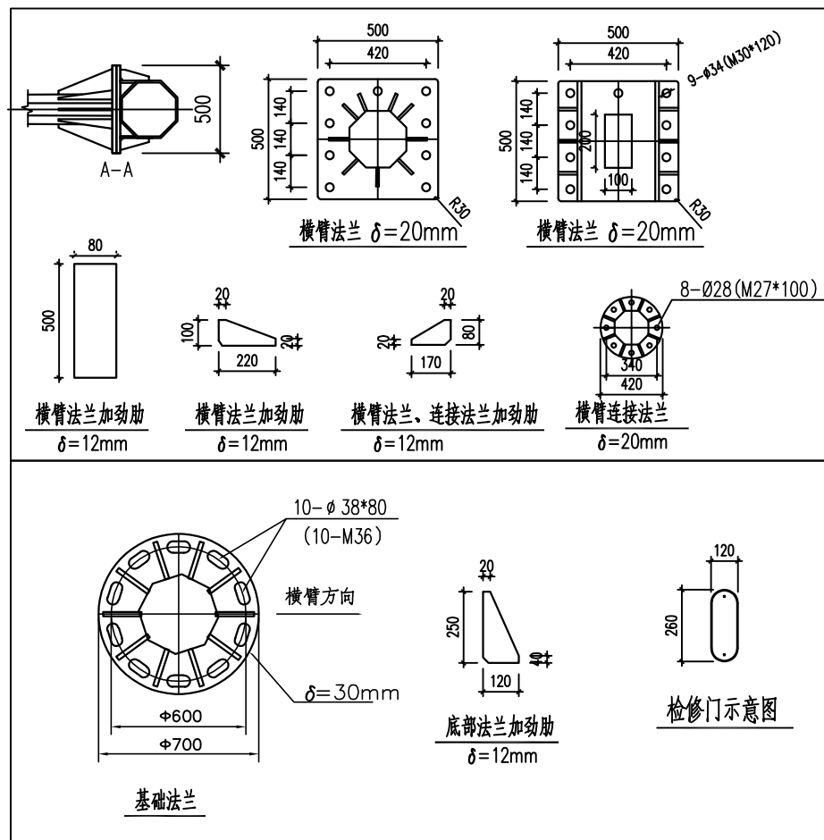
H7. 3L15米八角信号杆
