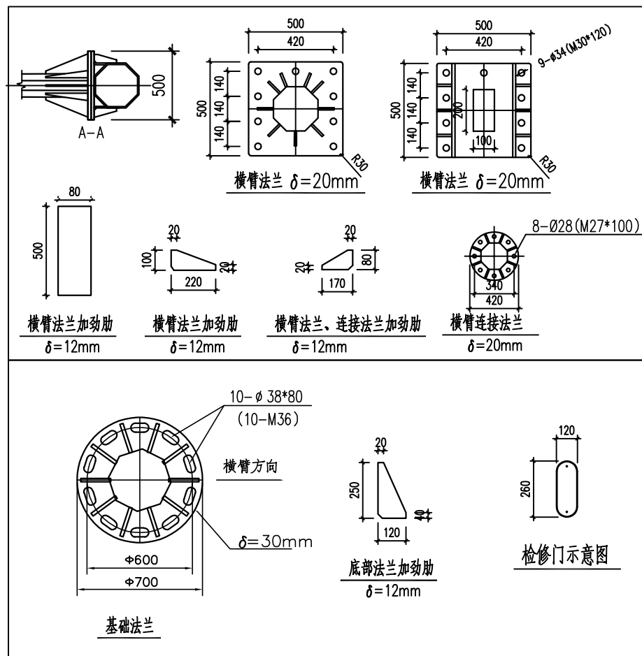
H6. 8L16米八角电警杆
