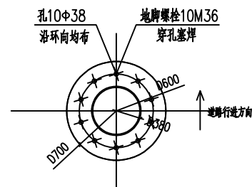
M-7 1:25 预埋钢板厚度为20mm 双螺母平行路沿石
