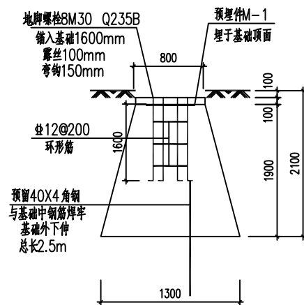
基础立面图
