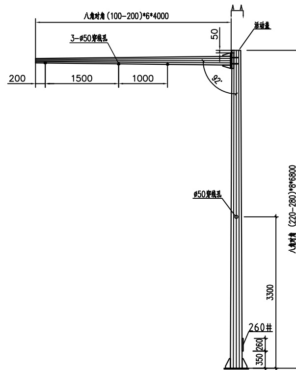
L=4m 杆件结构大样图
