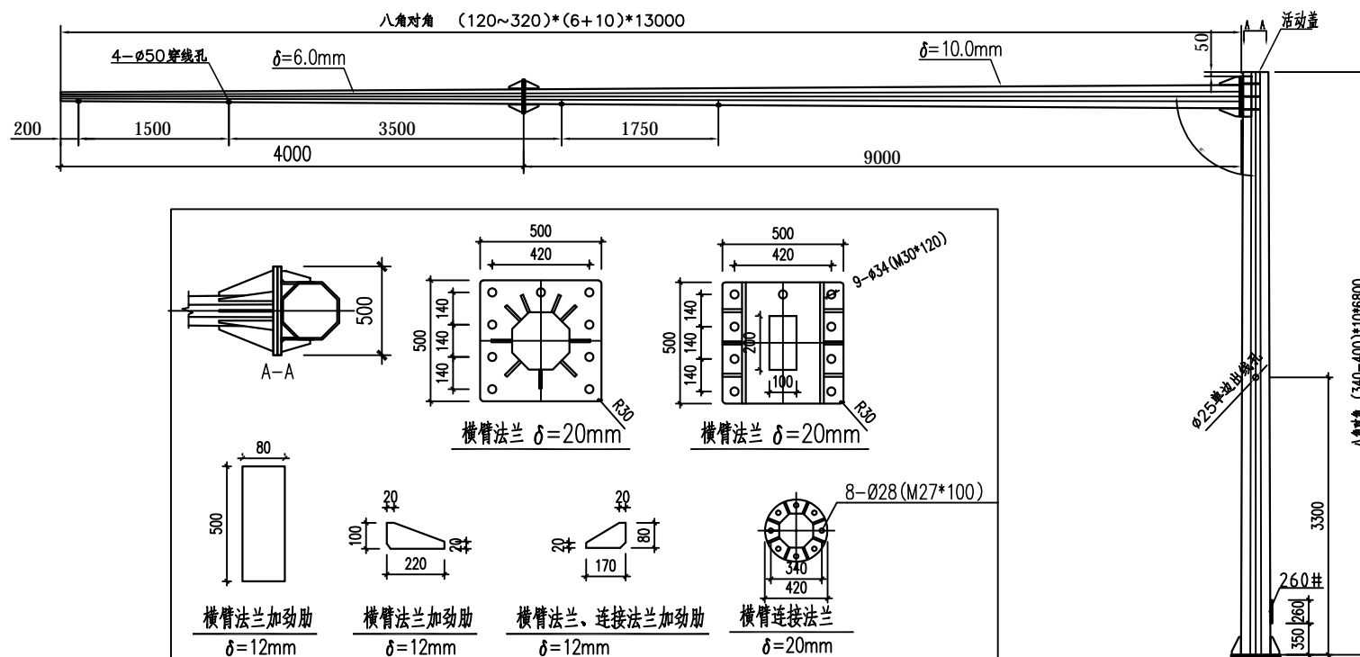
L=13m 杆件结构大样图
