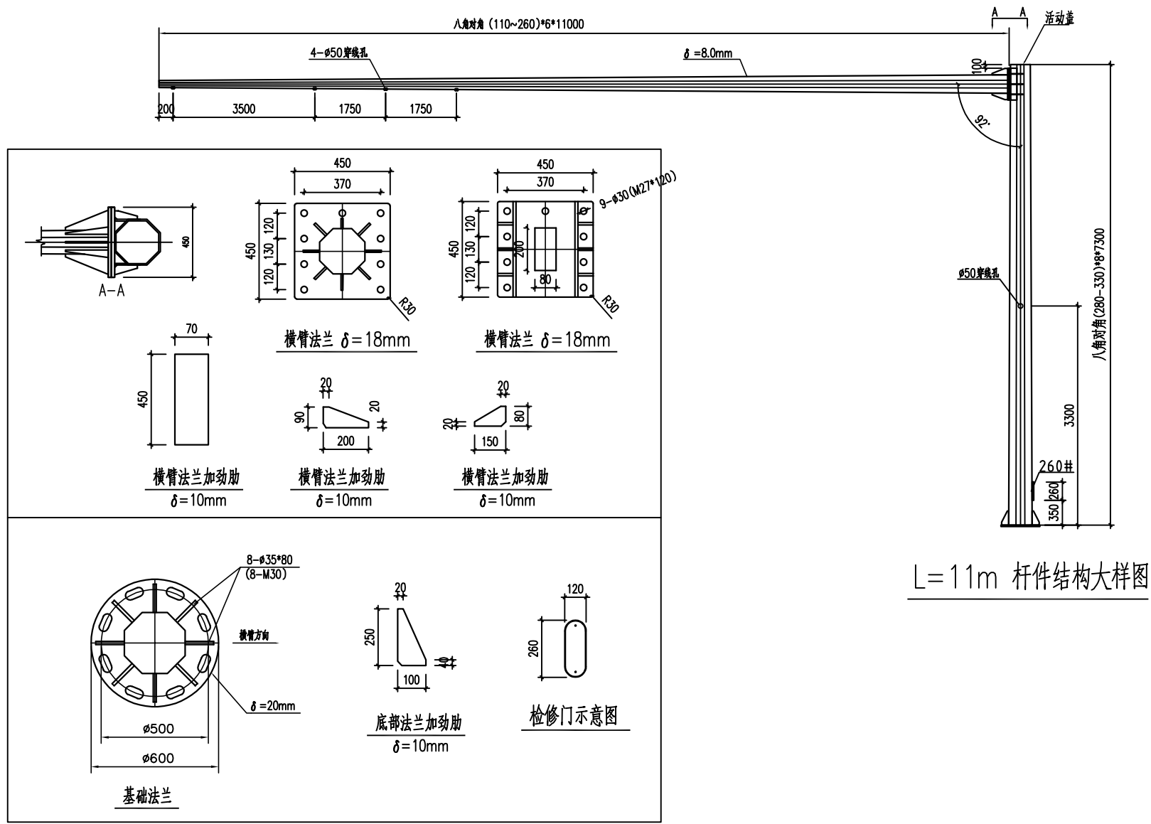
H7.3L11米八角信号杆
