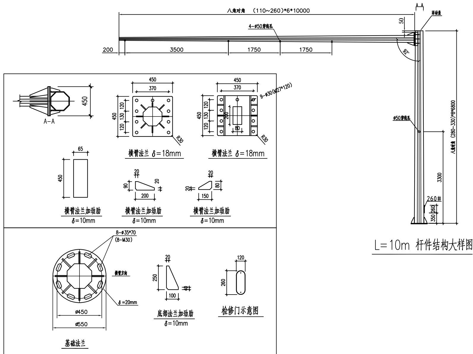
H6.8L10米八角电警杆
