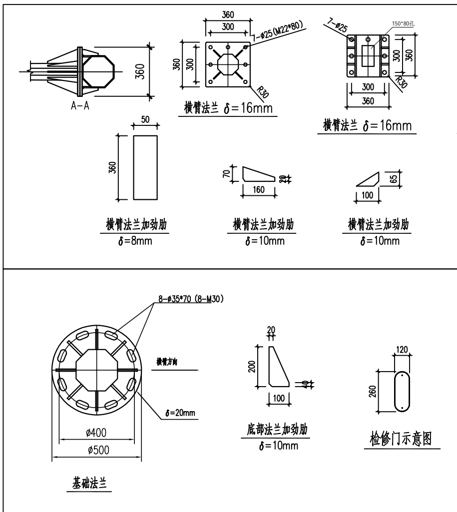
H6. 8L5米八角电警杆
