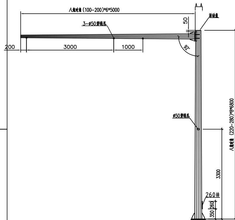
L=5m 杆件结构大样图
