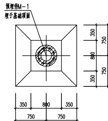
基础平面图
