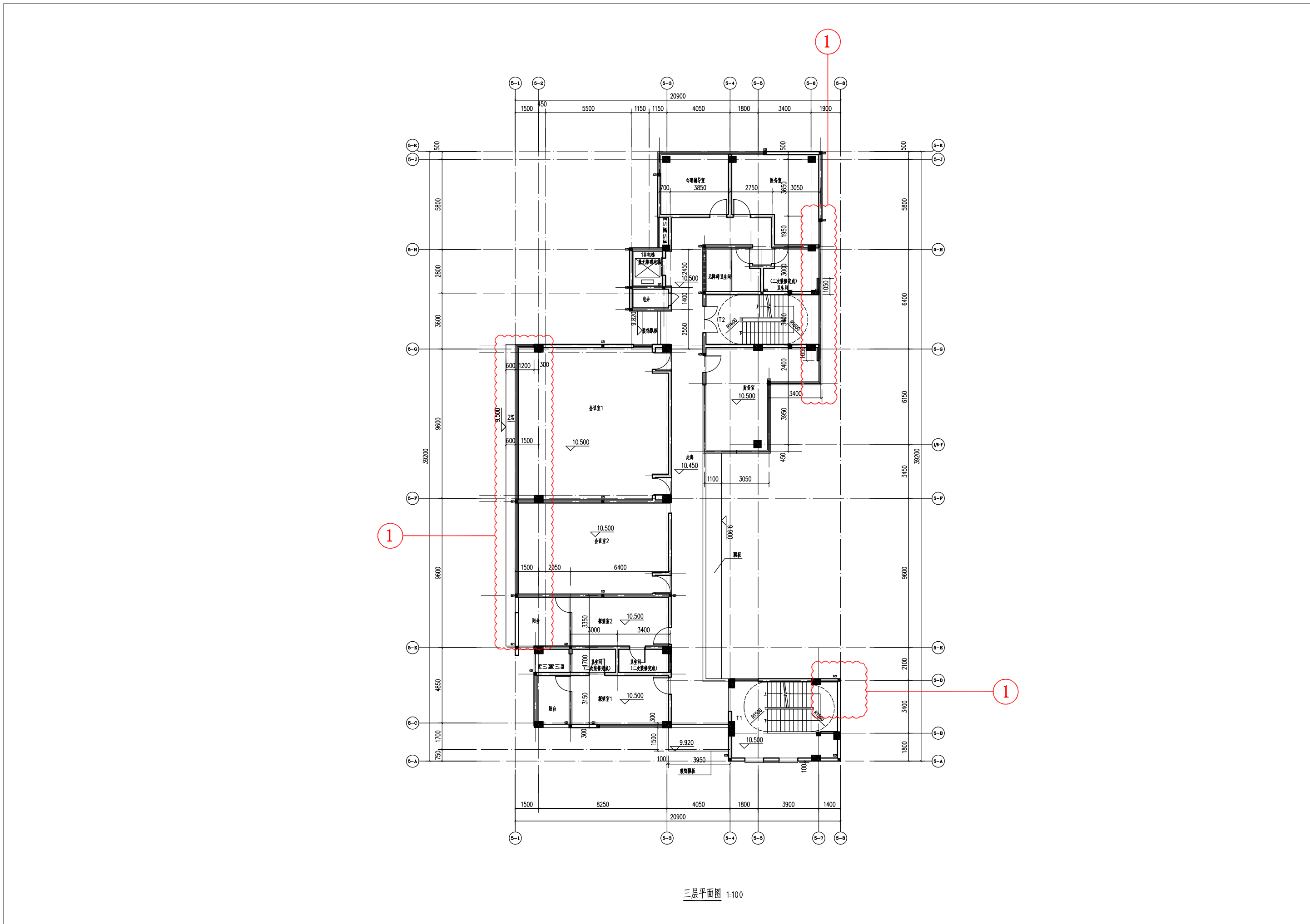
变更后的5栋 消防站三层平面图
