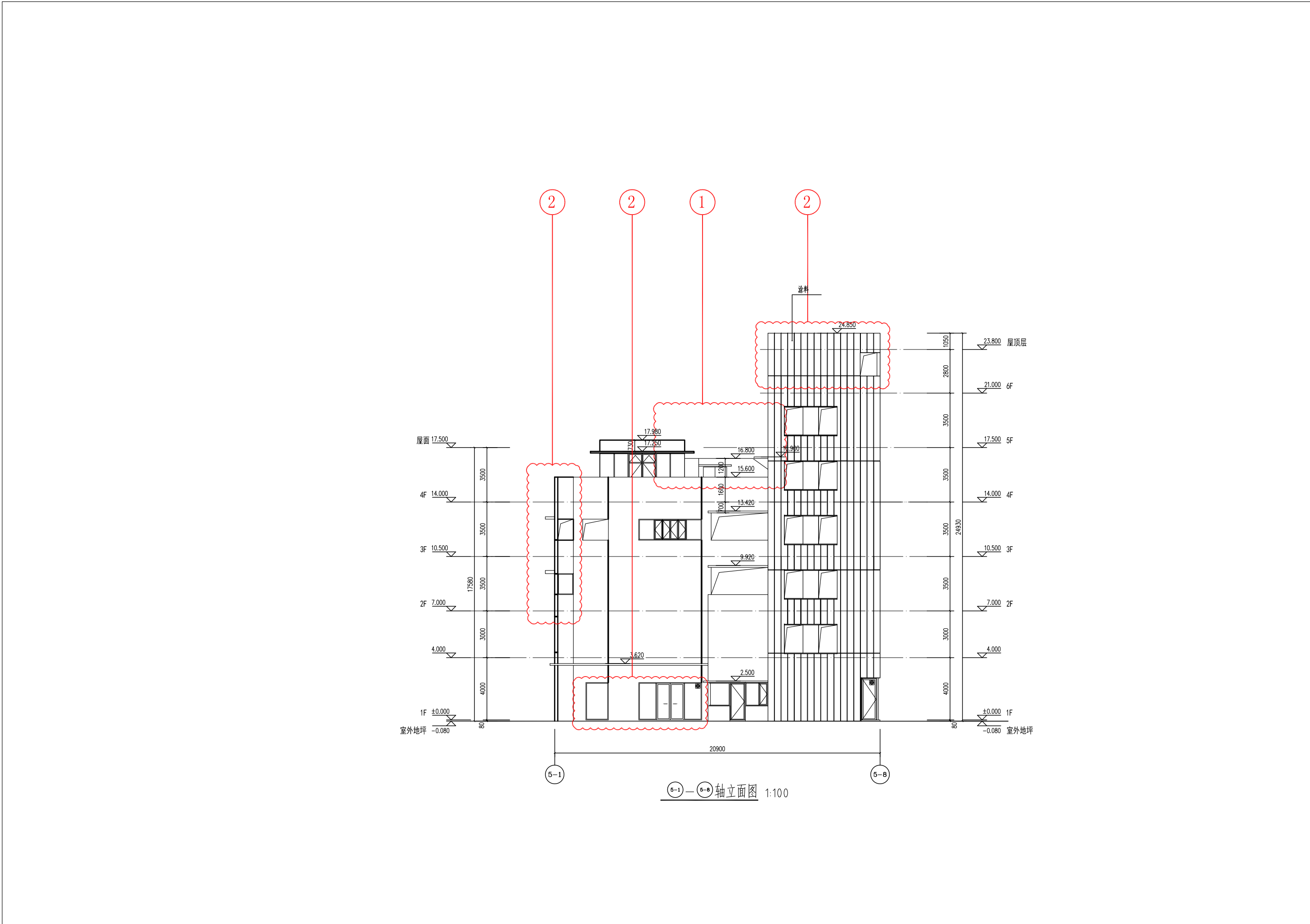
变更后的5栋 消防站 ⑤-1-⑤-8 轴立面图
