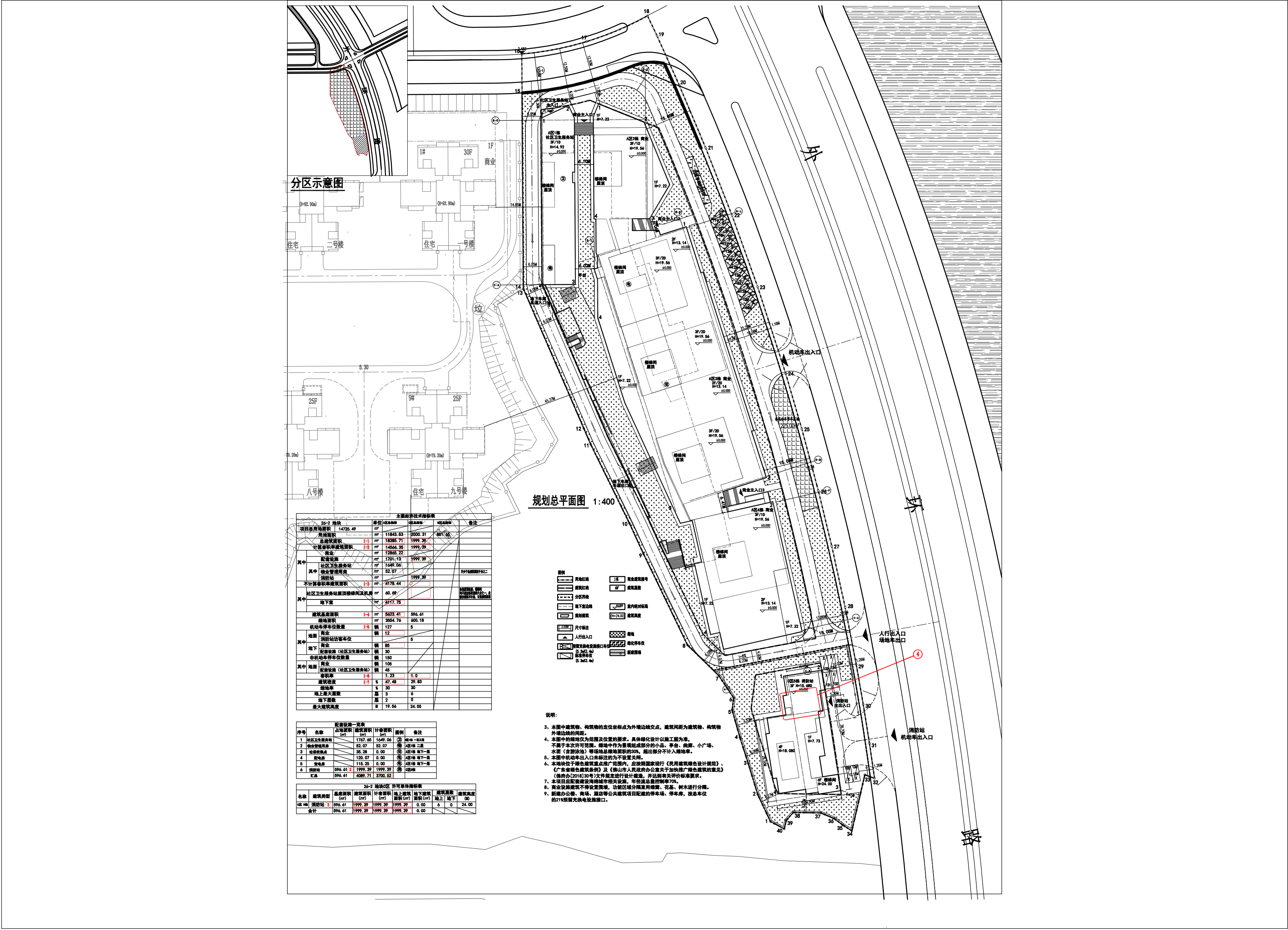
变更前的总平面图
