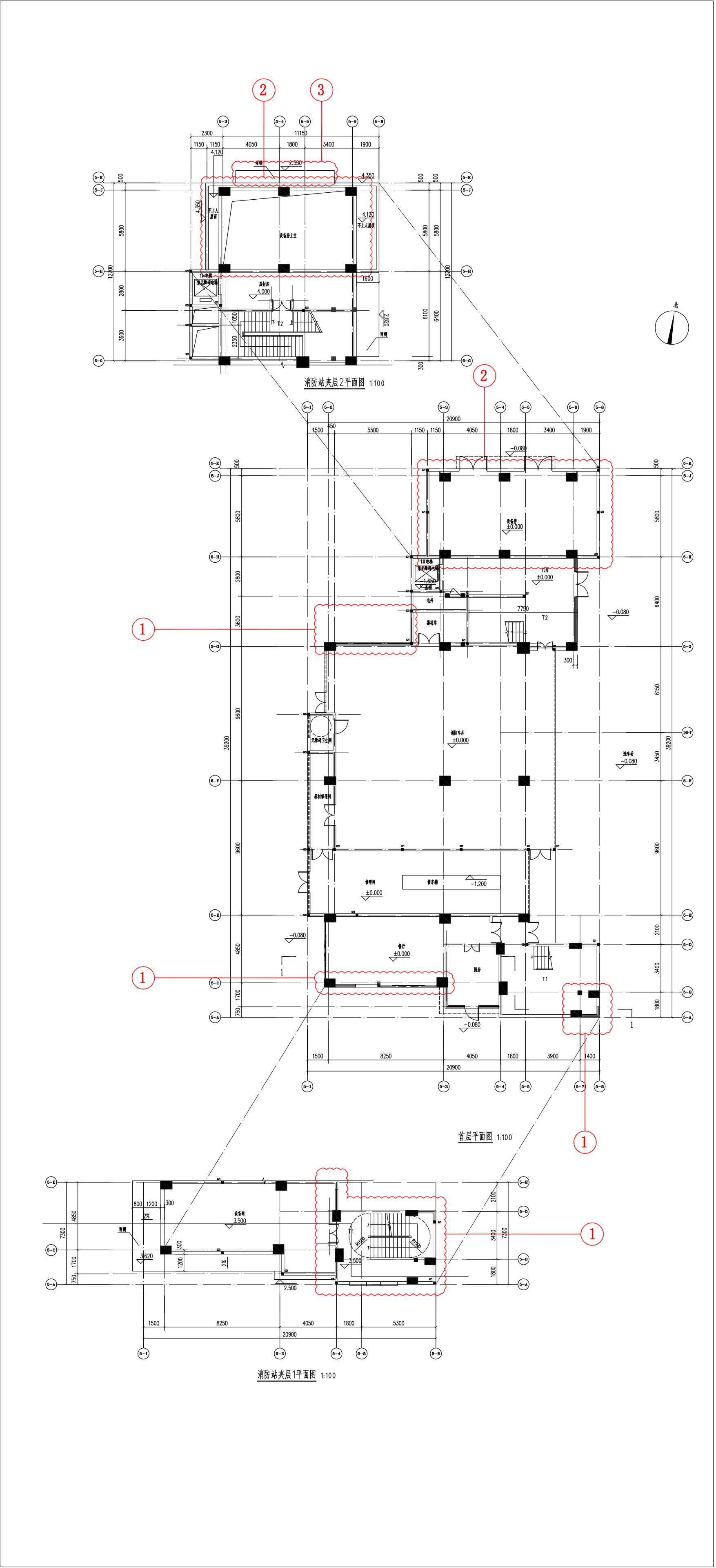
变更后的5栋 消防站首层、夹层平面图
