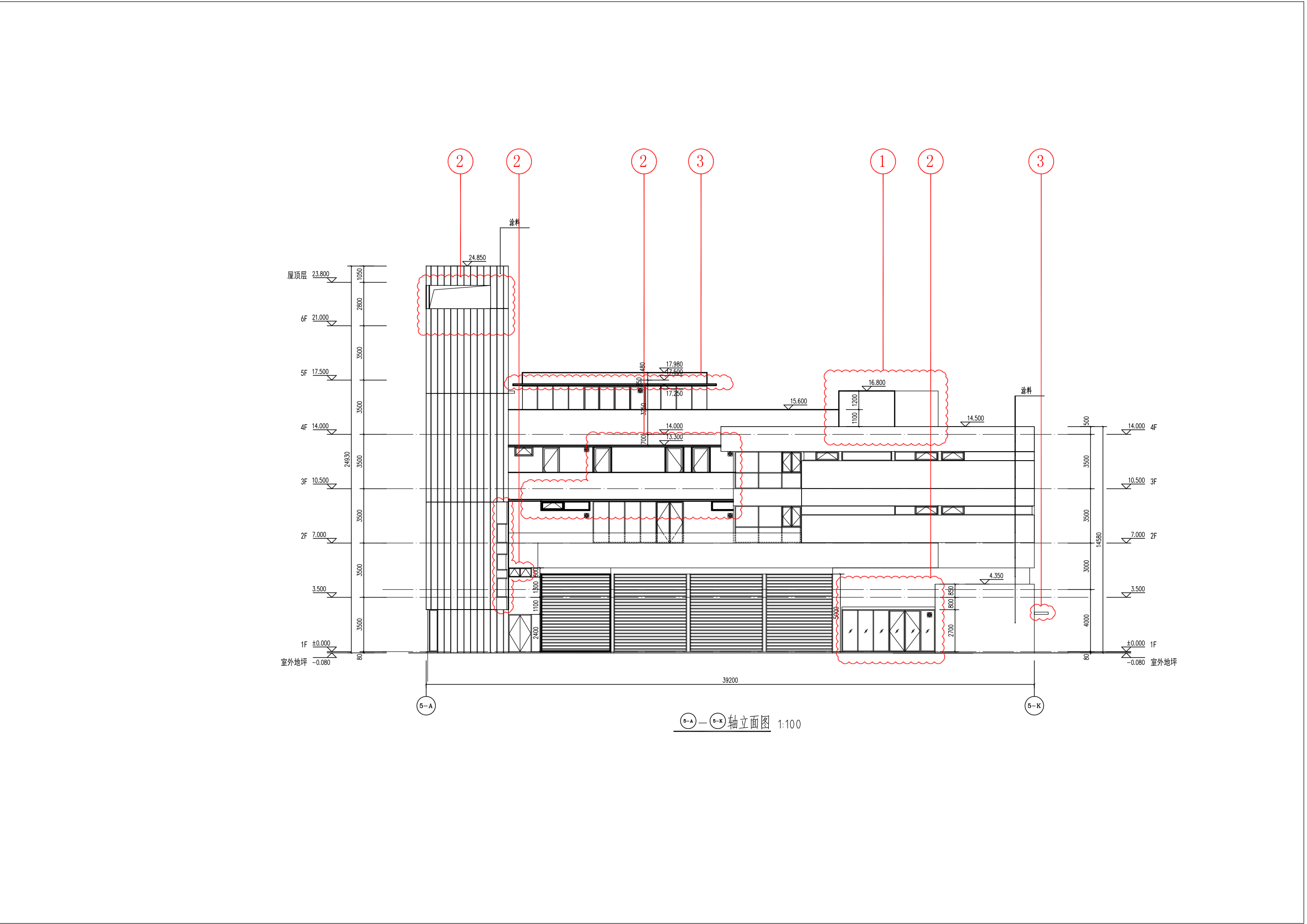
变更后的5栋 消防站 ⑤-A-⑤-K 轴立面图
