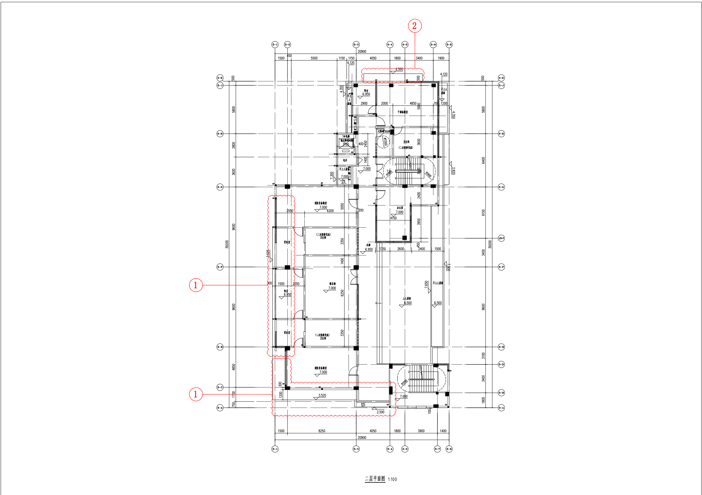
变更后的5栋 消防站二层平面图
