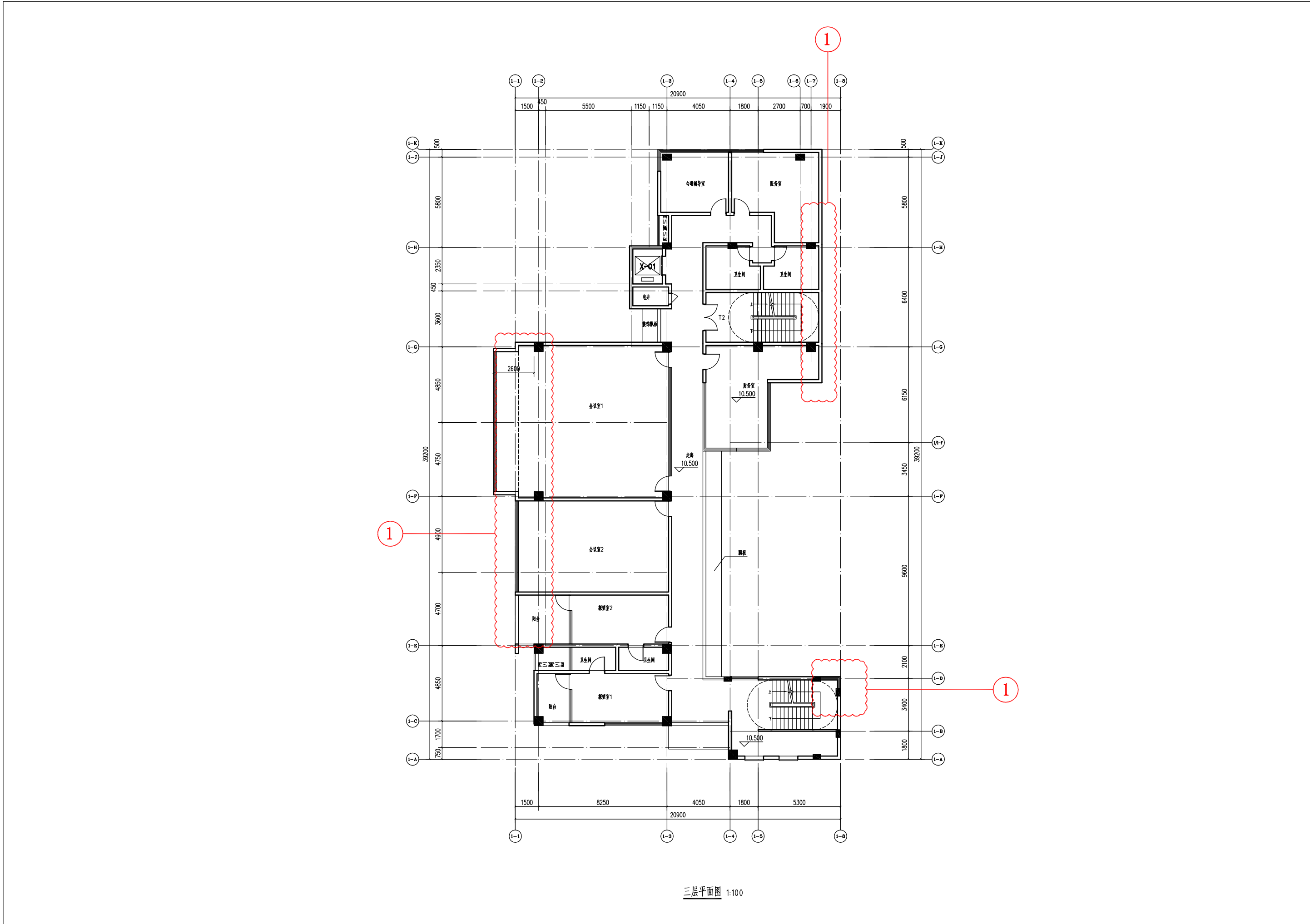
变更前的5栋 消防站三层平面图
