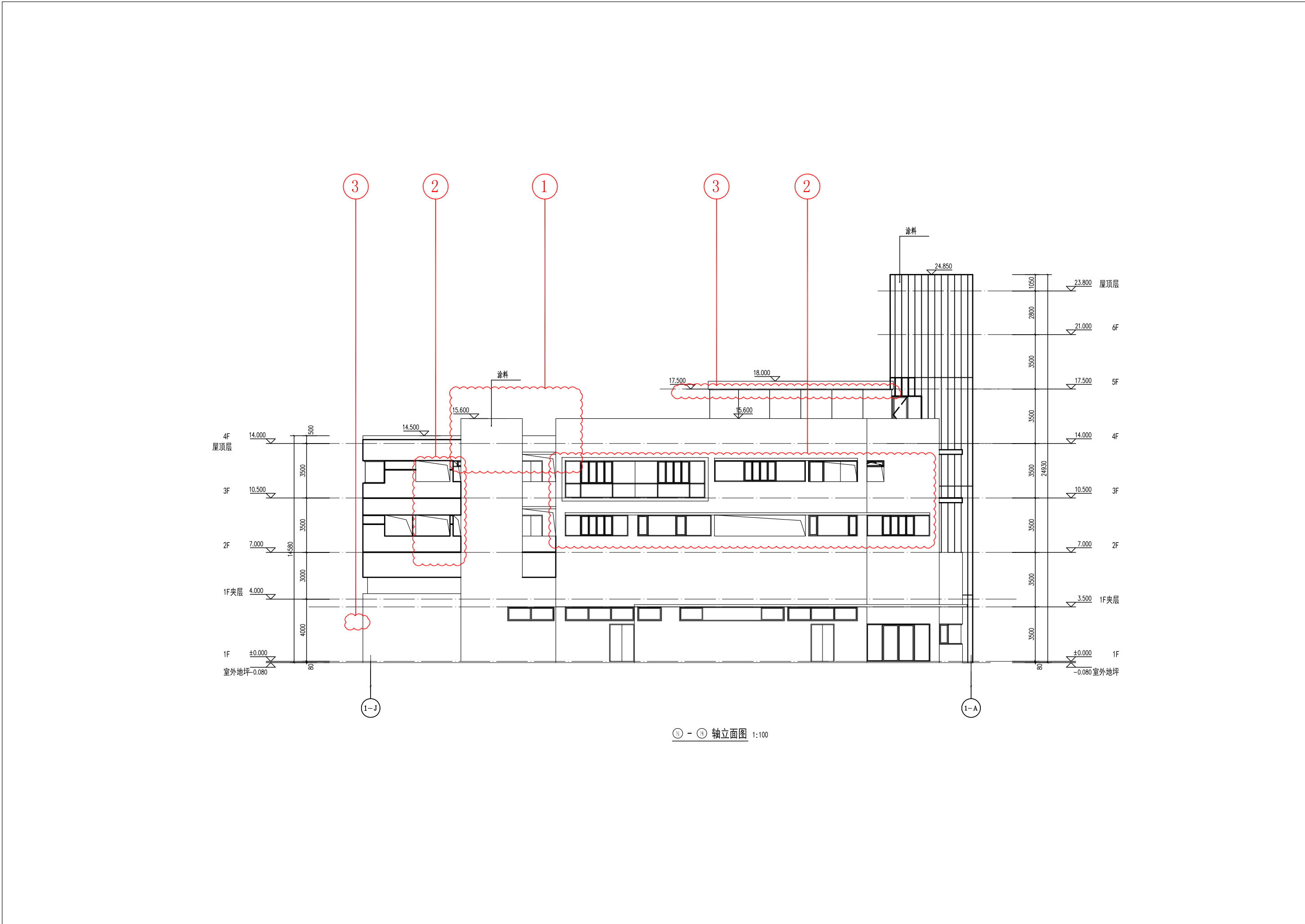
变更前的5栋 消防站 5-K-5-A 轴立面图
