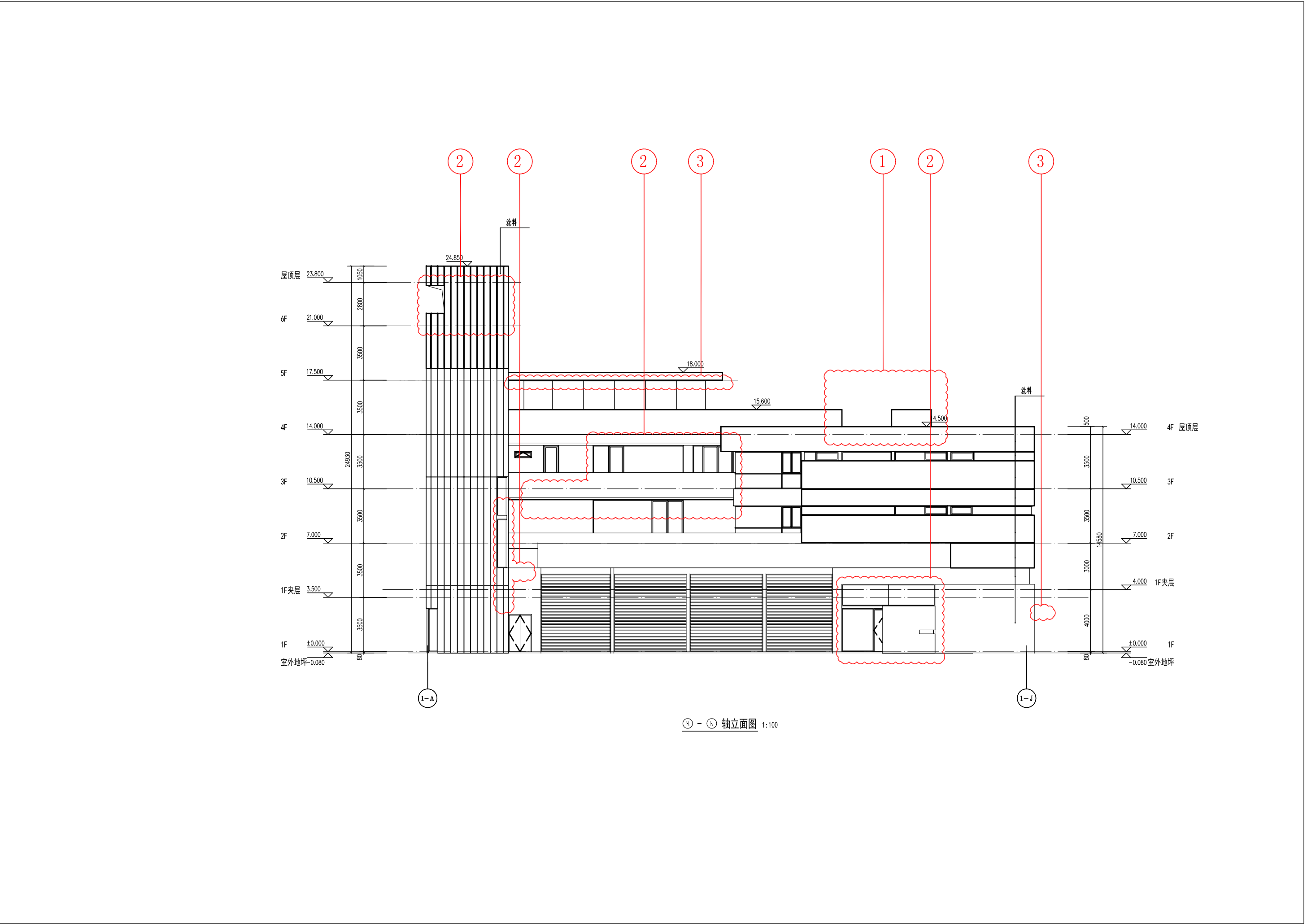
变更前的5栋 消防站 ⑤-A-⑤-K 轴立面图
