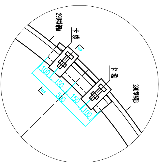
C放大图 (卡缆) 比例 1:10
