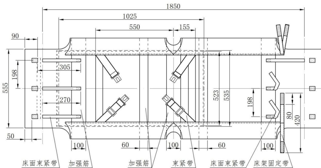
图 3 床背面结构及主要尺寸
