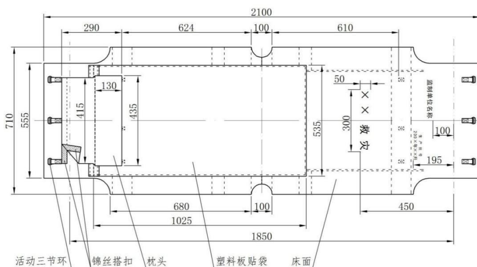
图 1 样式、结构及主要尺寸
