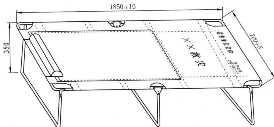
图 1 样式、结构及主要尺寸
