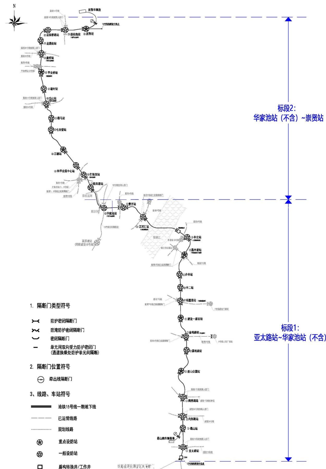
杭州地铁15号线一期人防设备招标区段划分示意图
