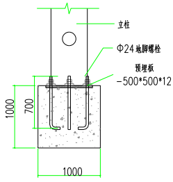
基础立面图
