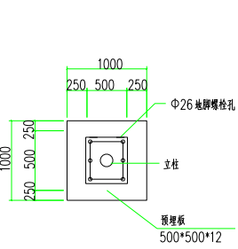
基础平面图
