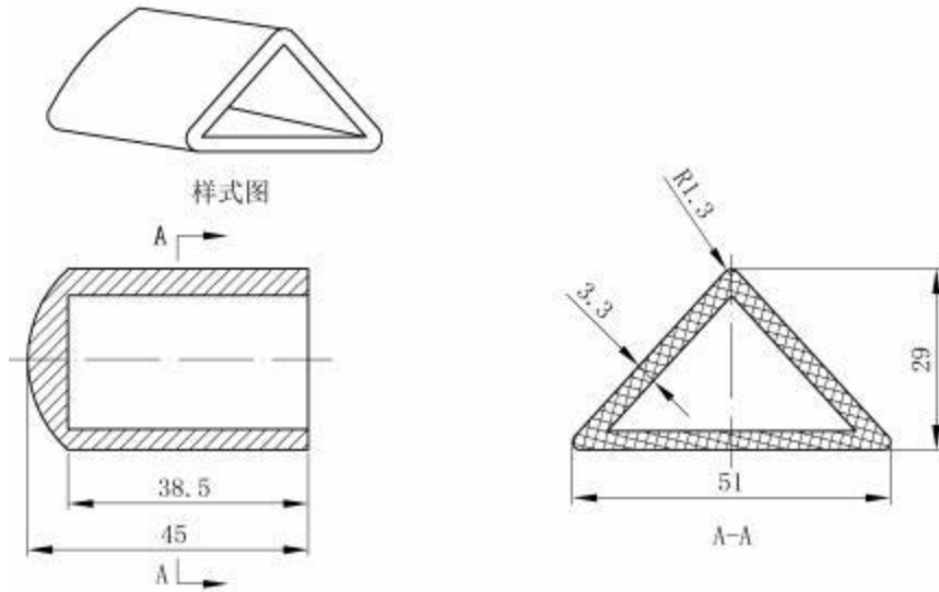
图C.6 橡塑桩头结构及主要尺寸
