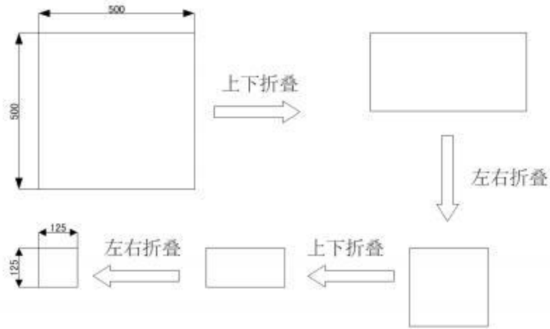
图L.1 试样折叠方法
