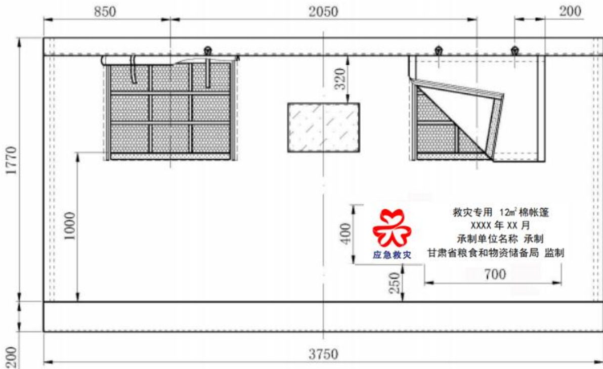
图A.7 篷体侧墙面结构及主要尺寸
