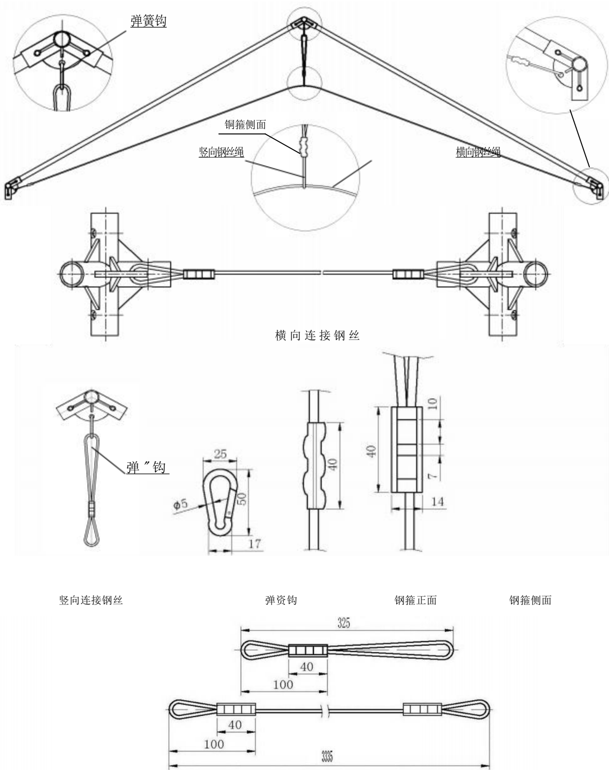
B.8 钢丝绳拉绳结构及主要尺寸
