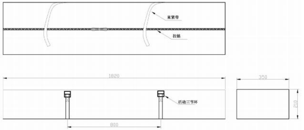
图A.20 一体化包装袋结构及主要尺寸
