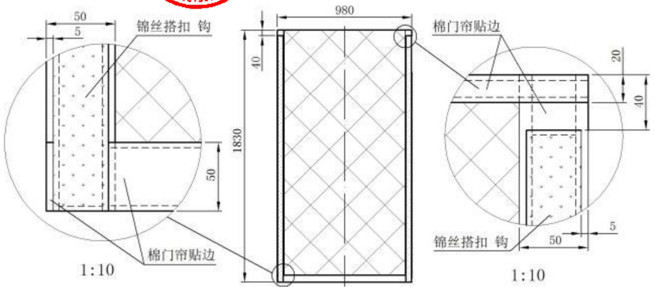
图A.19 棉内胆门帘结构及主要尺寸
