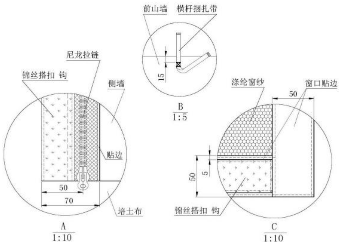
图A.8 篷体侧墙里结构及主要尺寸
