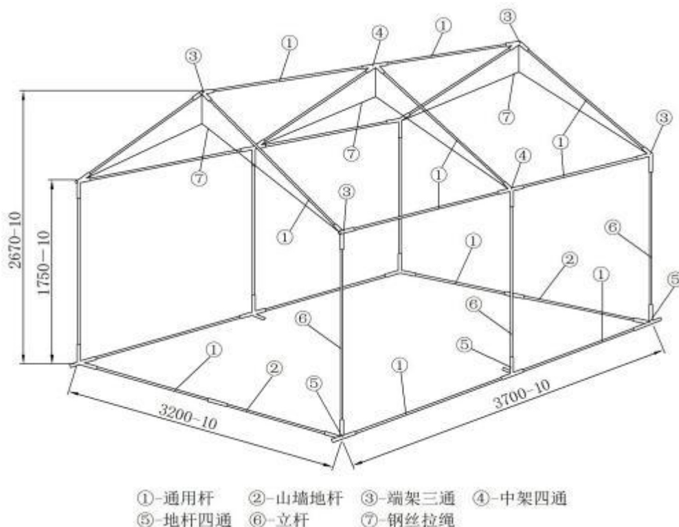
图 2 框架各部件名称、结构及主要尺寸
