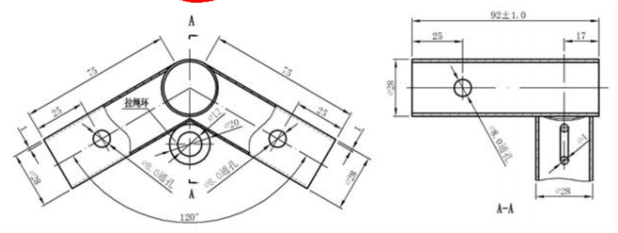
图B.4 端架三通结构及主要尺寸
