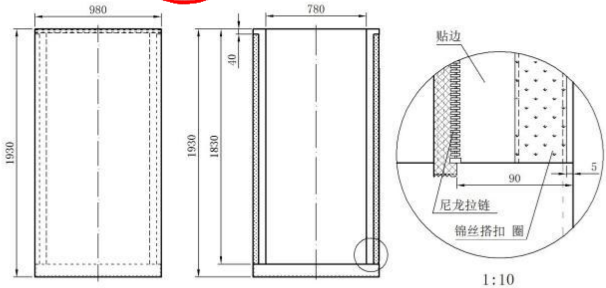
图A.6 单篷体门帘结构及主要尺寸
