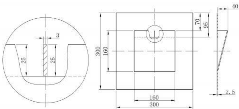
图C.5 风斗结构及主要尺寸
