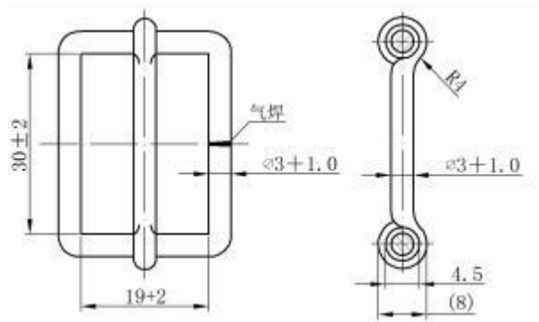
图C.3 活动三节环结构及主要尺寸
