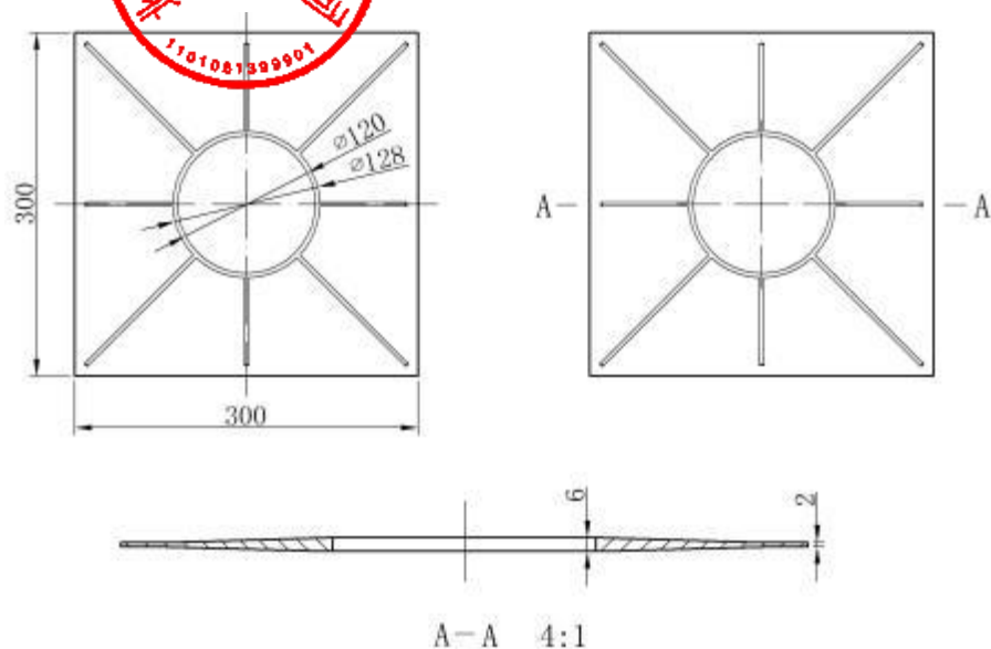
图C.4 烟囱口板结构及主要尺寸
