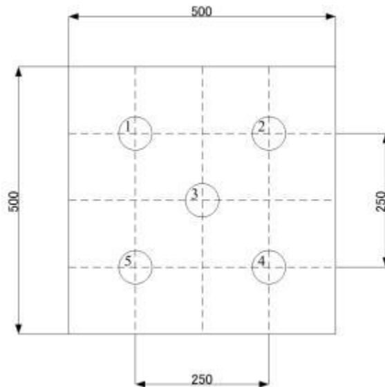
图L.2 试样静水压测点位置
