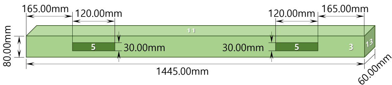
图 1 堵塞尺寸示意图
