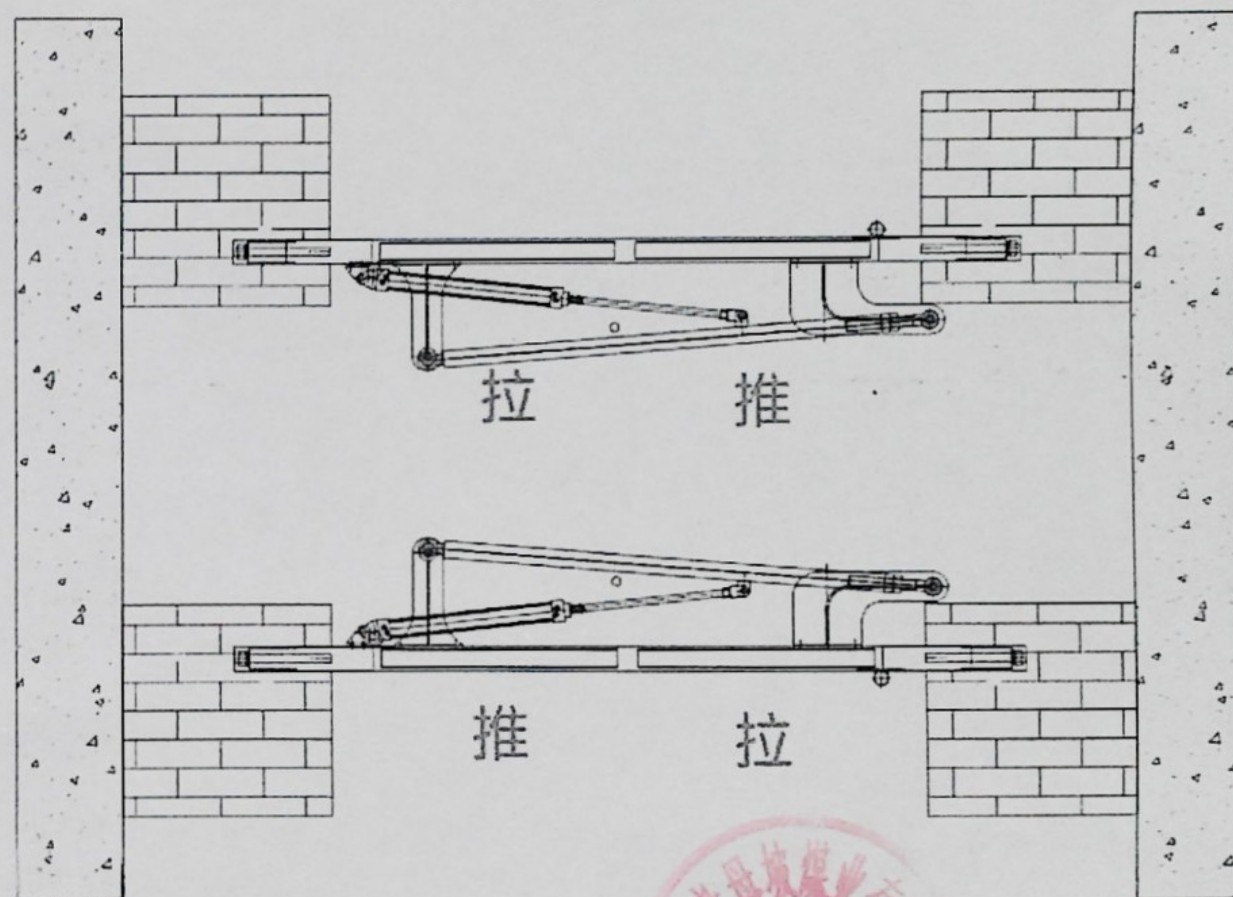
安装示意图
