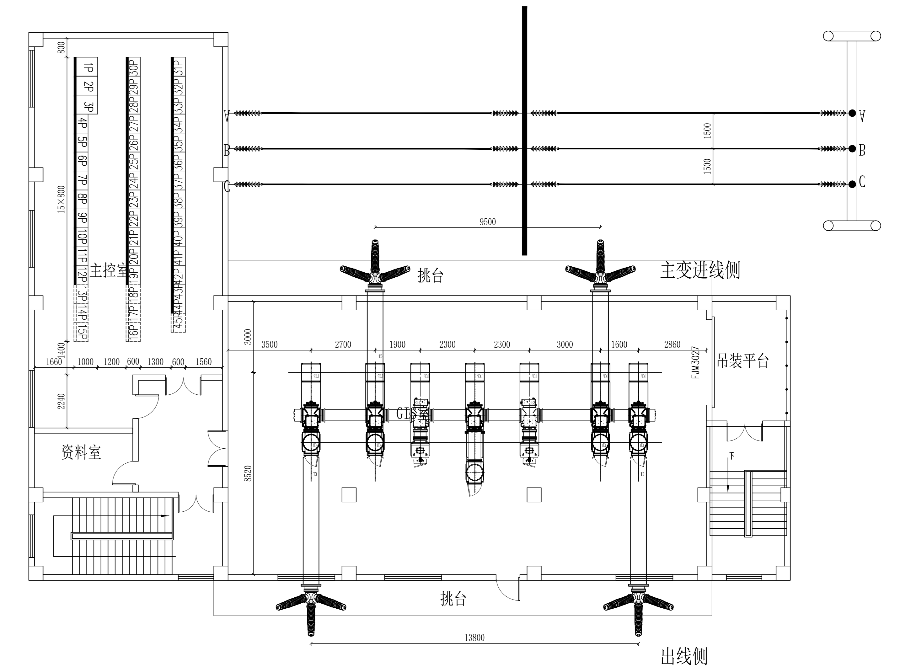
4.8m平面布置图
