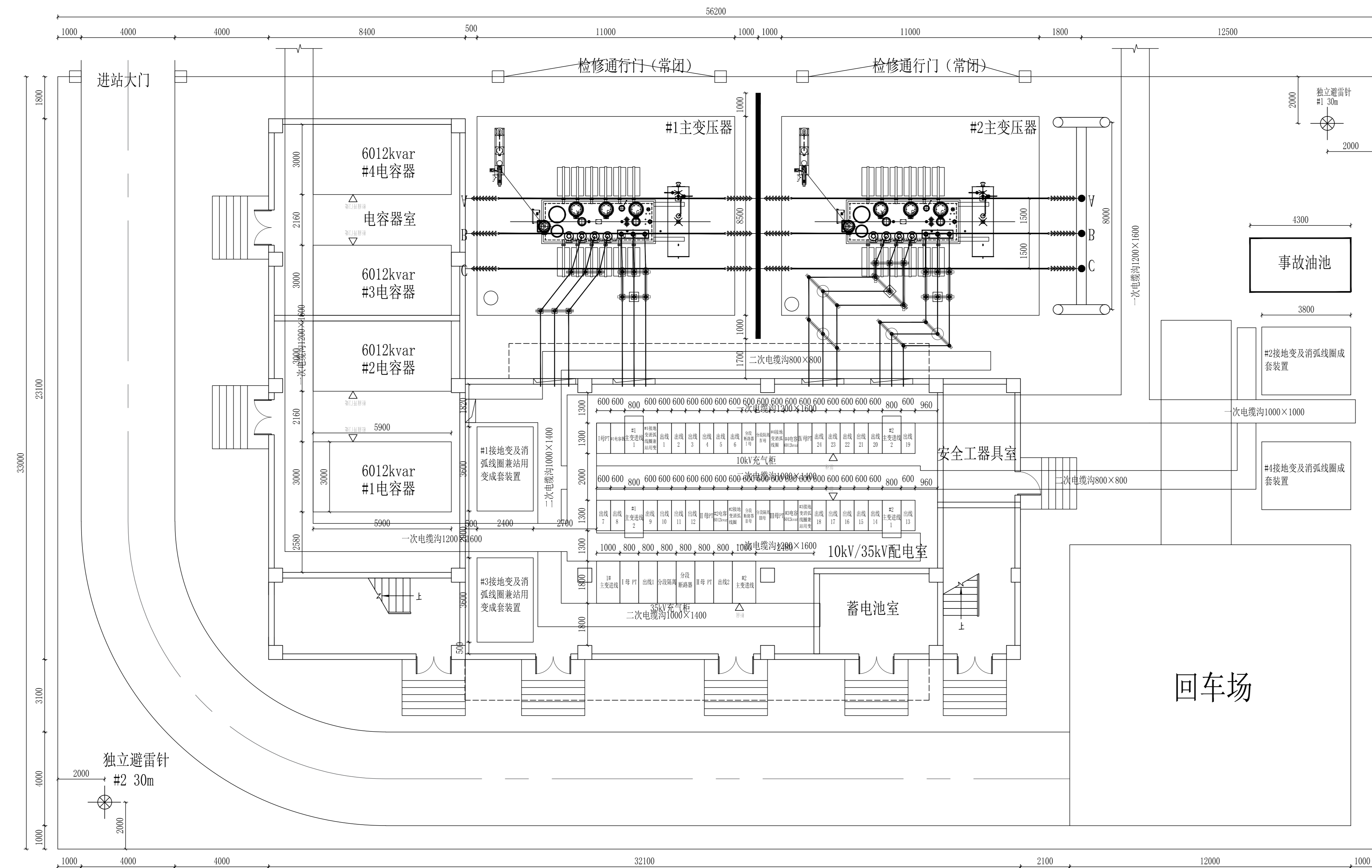
0.0m平面布置图
