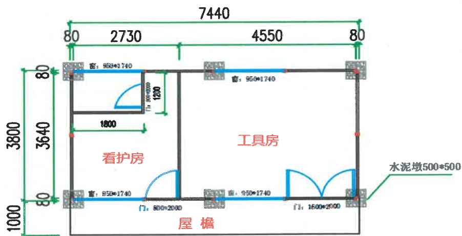
2K*4K*3P(平面图)
